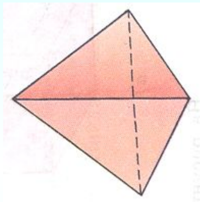
тетраэдр
