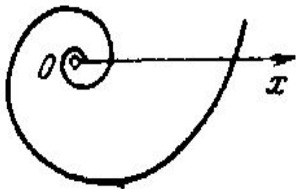
Рис. 101. логарифмическая СПИРАЛЬ
