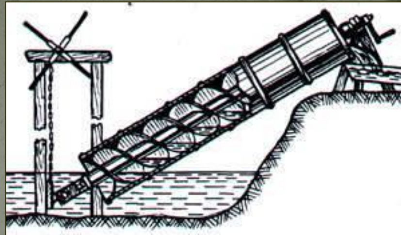
Архимедов винт - водонапорная машина.
