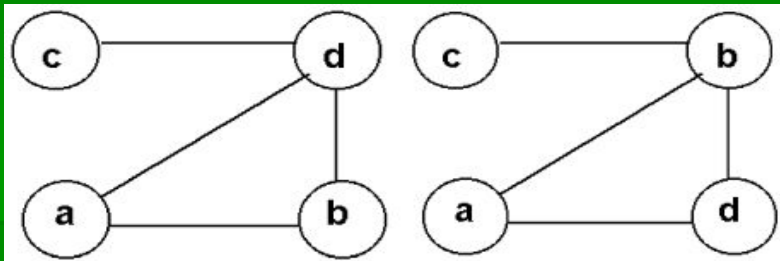
Рис. 2. Пример двух разных графов
