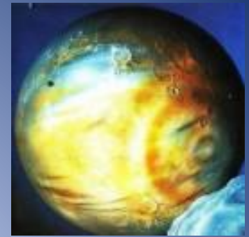
Pluto
