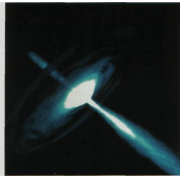
Черная дыра, окруженная аккреционным диском. Вдоль осей вращения диска формируются мощные выбросы электронов и субатомных частиц (джеты).
