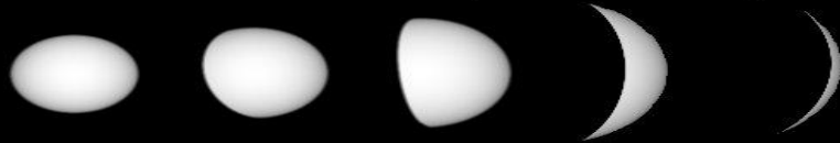
Фазы Меркурия
