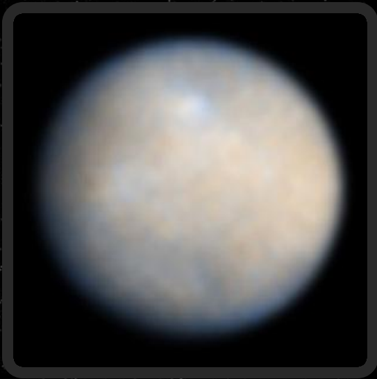
Церера
