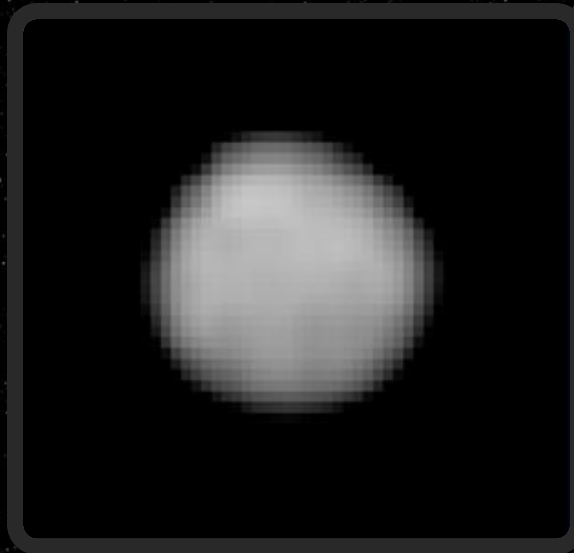
Паллада
