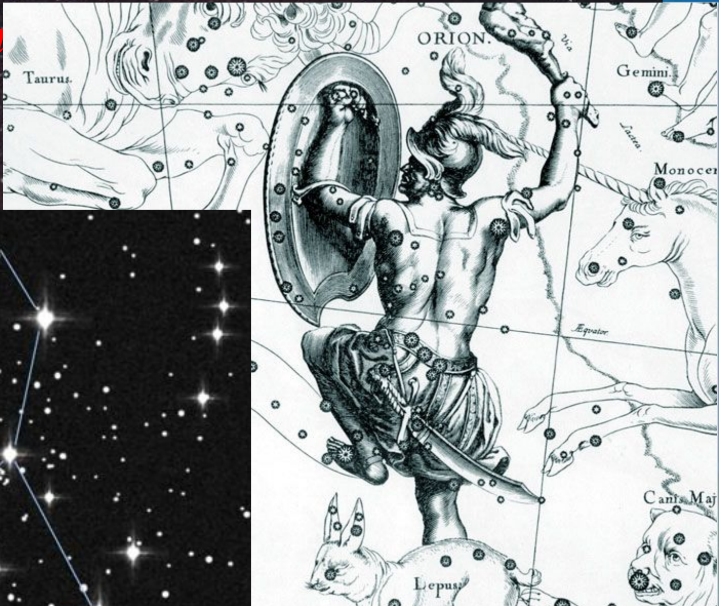
Созвездие Ориона
