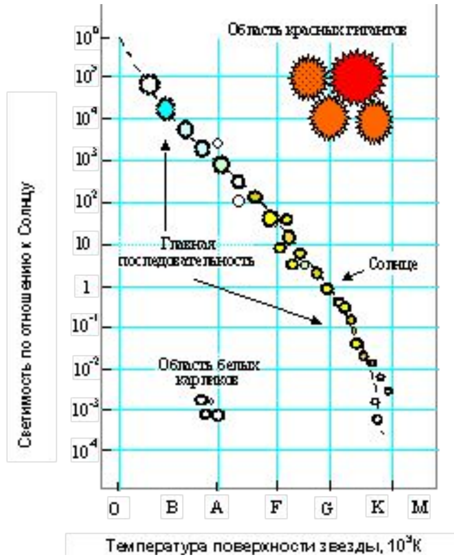
Диаграмма Герцшпрунга-Рессела
