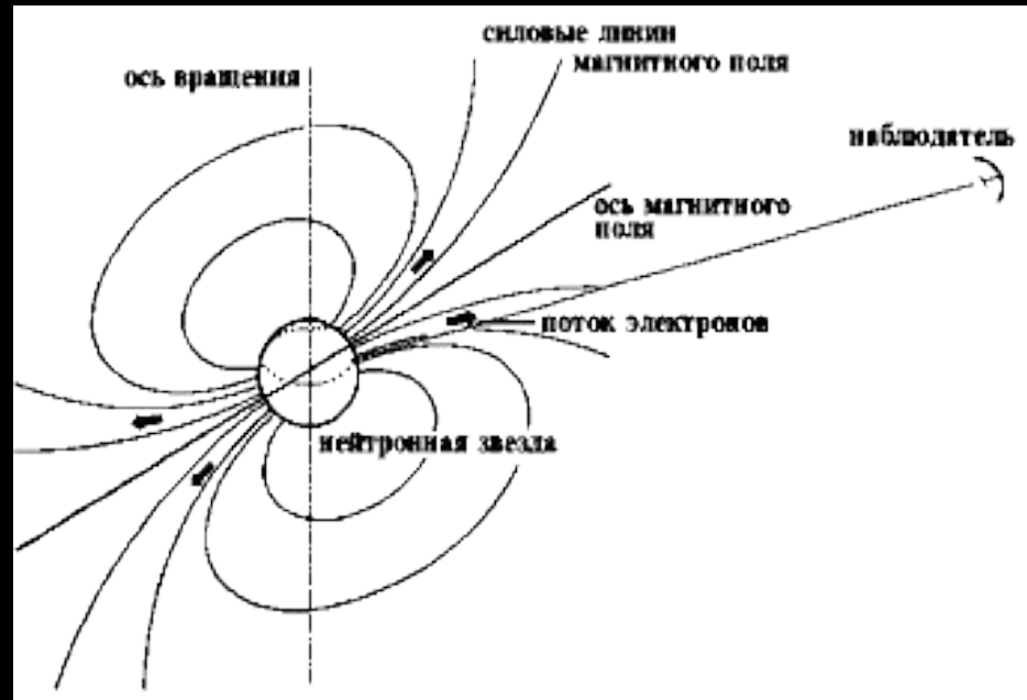
Модель пульсара
