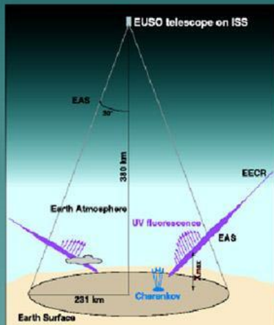
Рис. 12. Детектирование ШАЛ из космоса.
