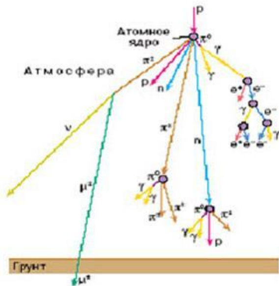
Рис. 5. Схема ядерно-каскадного процесса в атмосфере. В результате соударения протона космических лучей с ядром атома воздуха образовались \pi^0 - и \pi^- -мезоны. \pi^0 -Мезон породил электронно-фотонный ливень (показан в правой части рисунка). \pi^- -Мезоны генерировал новый \pi^0 -мезон и заряженные \pi^- -мезоны второго поколения, часть \pi^- -мезонов распалась, породив мезоны. Протон очень высокой энергии способен породить в атмосфере Земли десятки поколений и образовать миллионы и миллиарды вторичных частиц, генетически связанных между собой, — так называемые широкие атмосферные ливни
