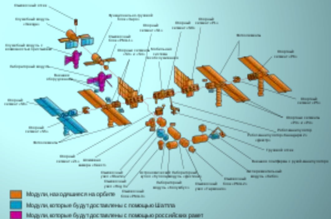
Сборка МКС на октябрь 2008 года
