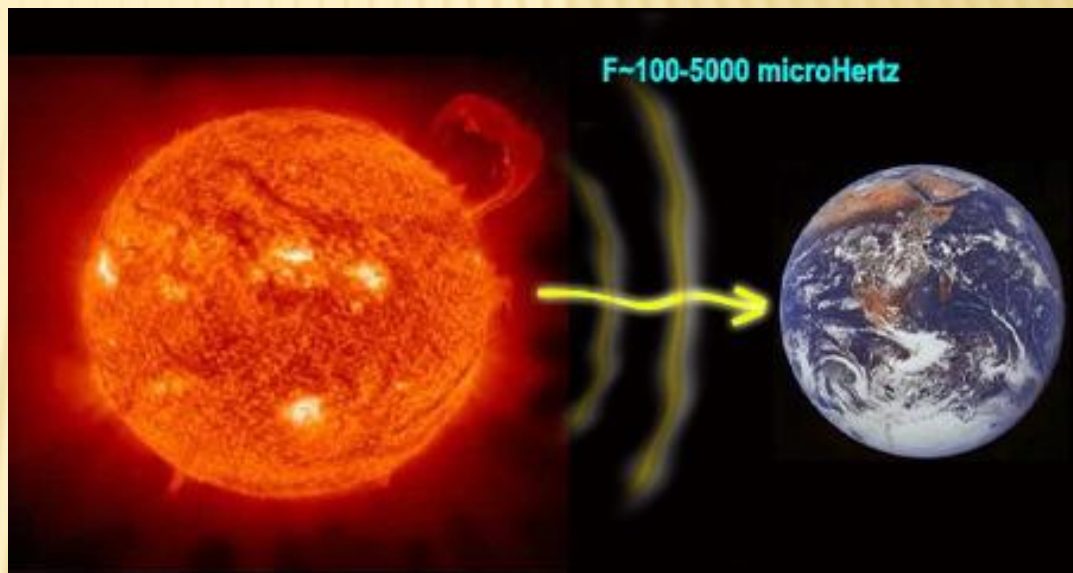
"Солнечный Гольфстрим": влияние Солнечных бурь на Землю
