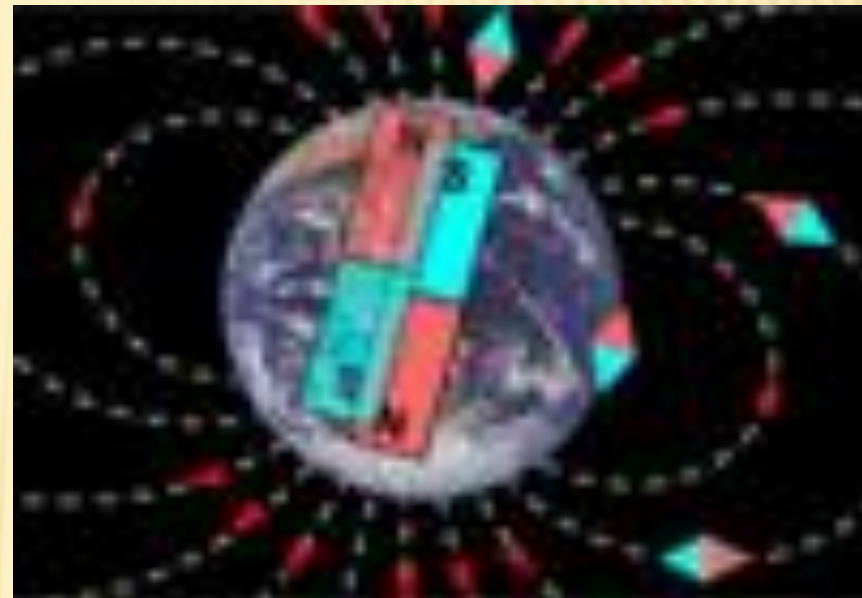
Смена полюсов на Земле
