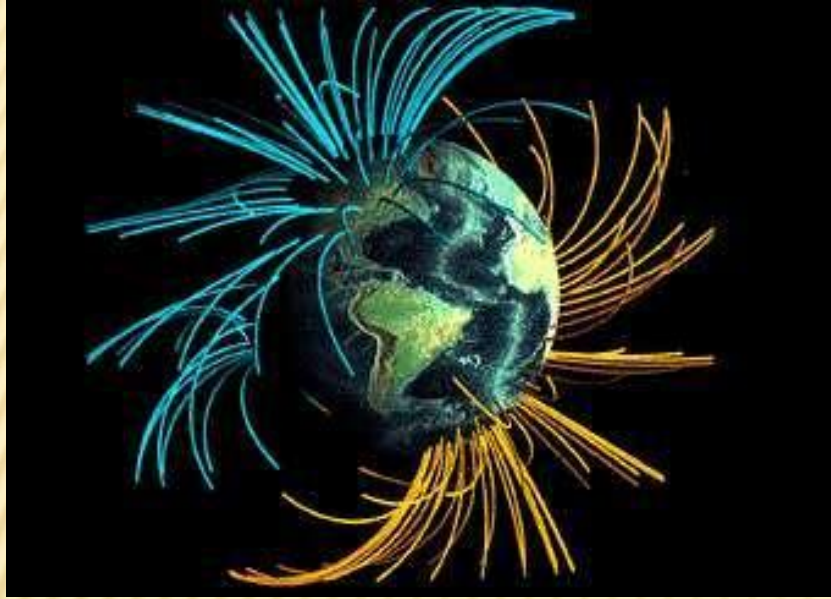
Магнитные полюса Земли: северный и южный
