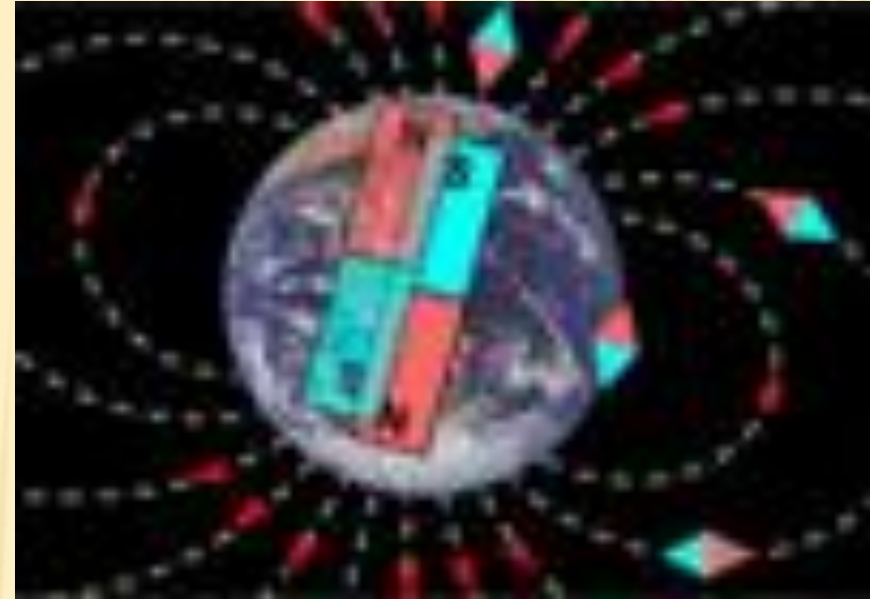
Смена полюсов на Земле
