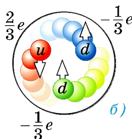
Кварковая структура нуклонов а) протон; б) нейтрон
