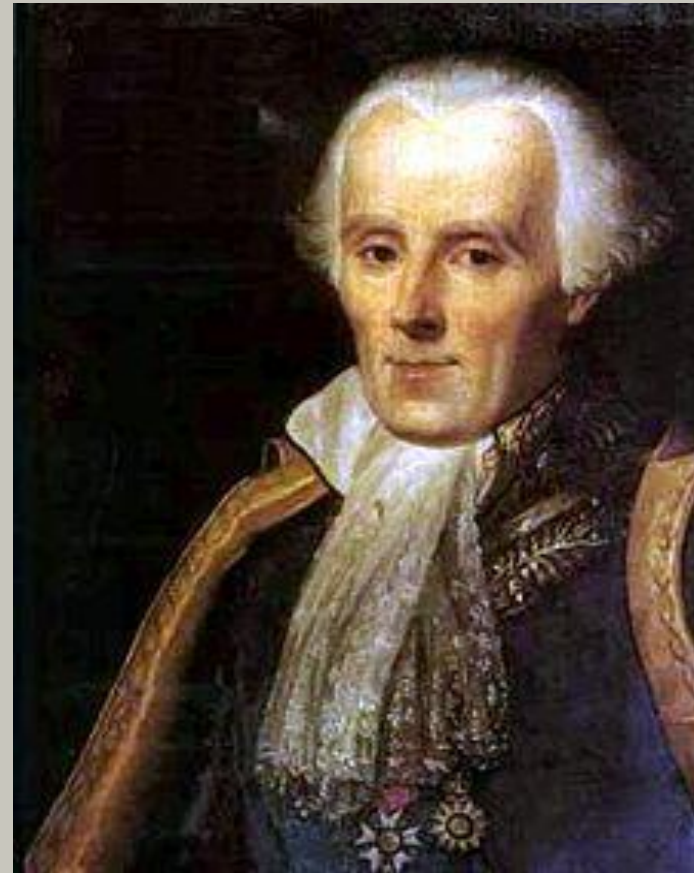
Лаплас
