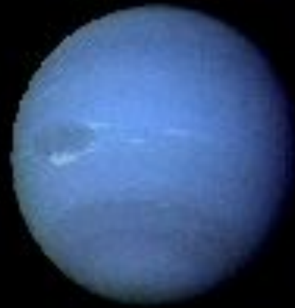
Нептун
