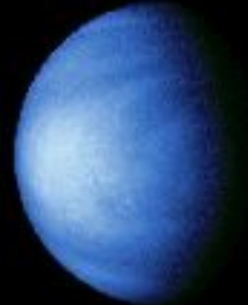
Венера
