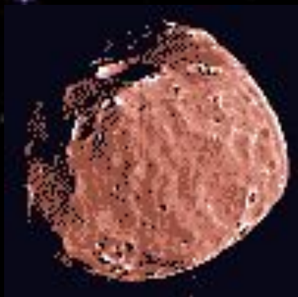
Фобос
