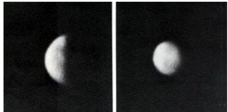
Лучшие фотографии Меркурия с Земли.
