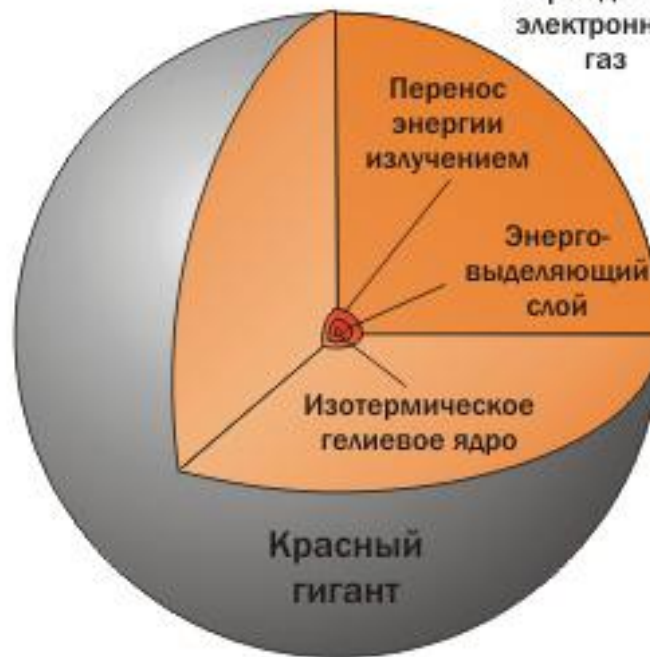
Вырожденный электронный газ
