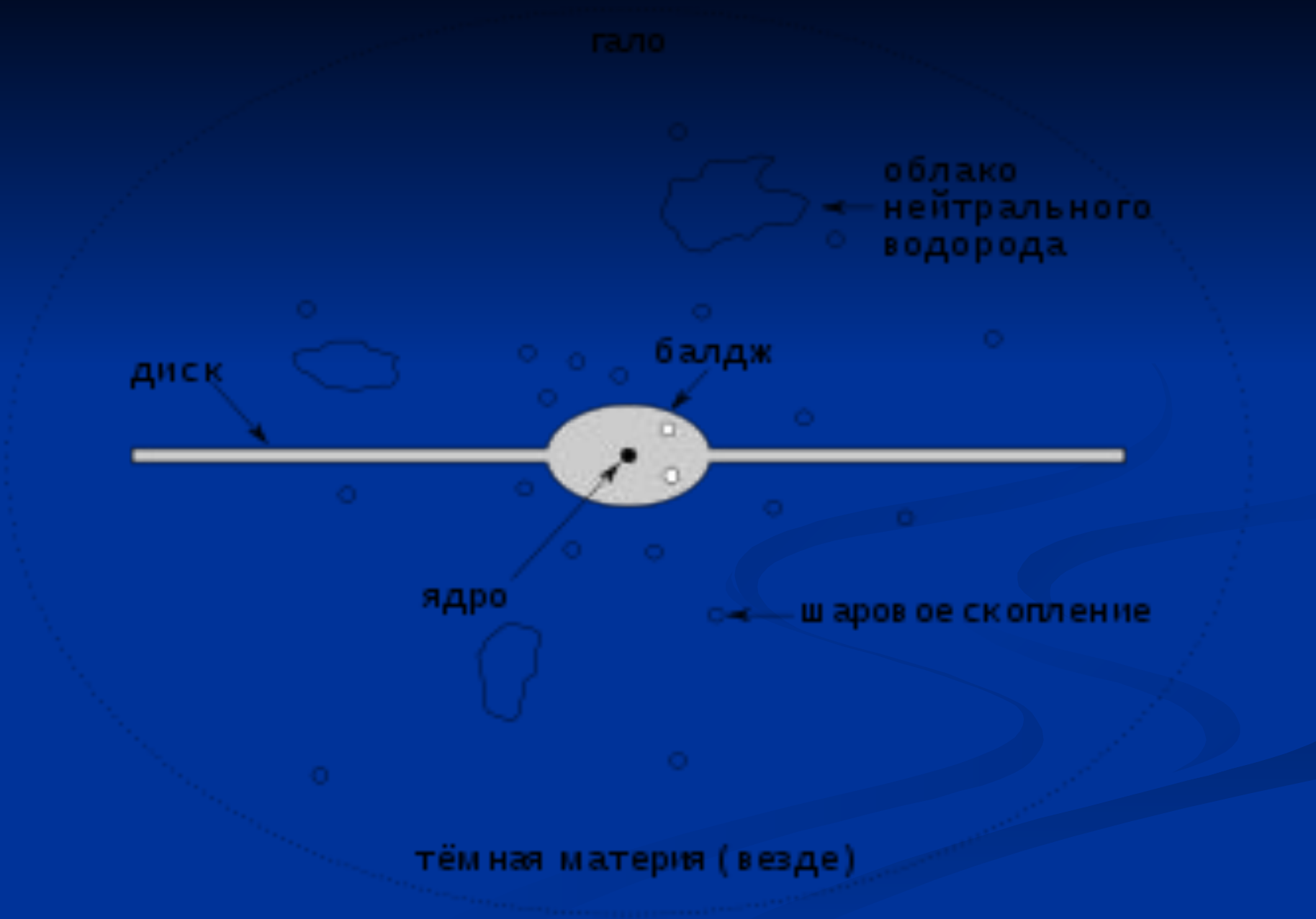
Схема спиральной галактики, вид в профиль
