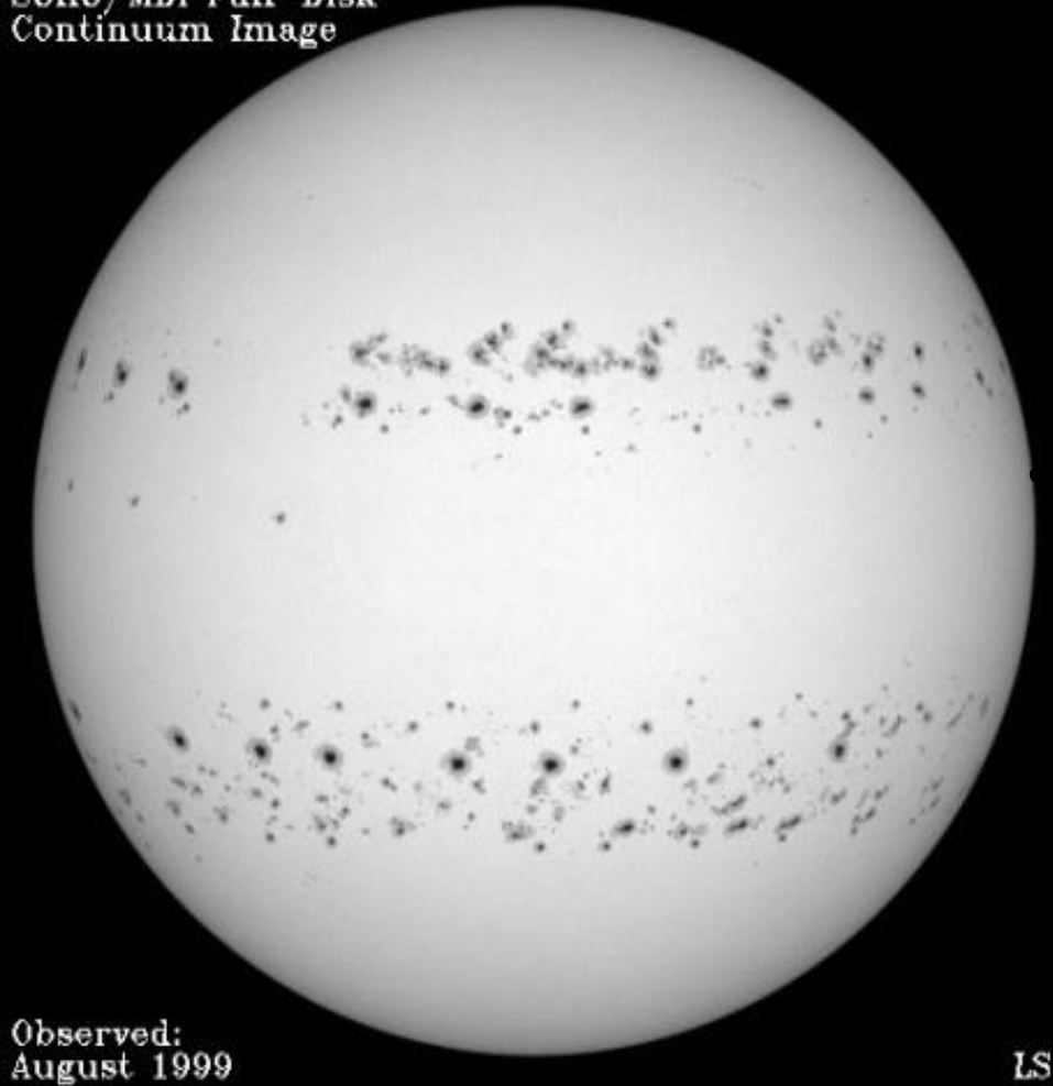
Солнечные пятна
