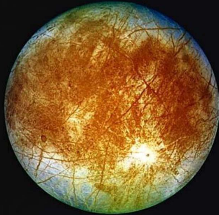
Европа, спутник Юпитера
