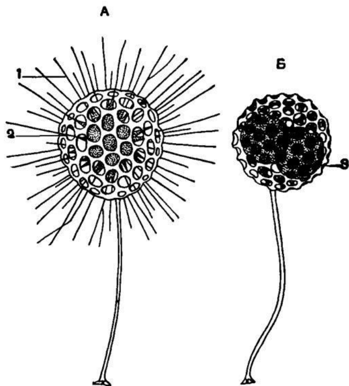
Рис. 39. Солнечник Clathrulina elegans : 1 — аксоподии; 2 — скелет, 3 — дочерние особи внутри скелета материнской особи.
