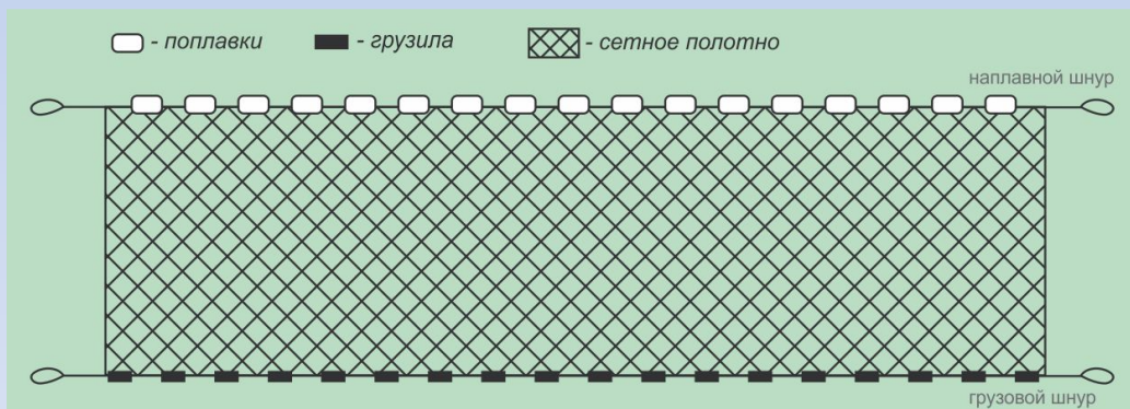
Плавные сети
