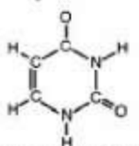
УРАЦИЛ [U]
