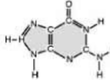
[G] ГУАНИН
