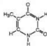
[T] ТИМИН
