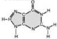
ГУАНИН [G]
