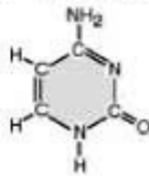
[G] ГУАНИН
