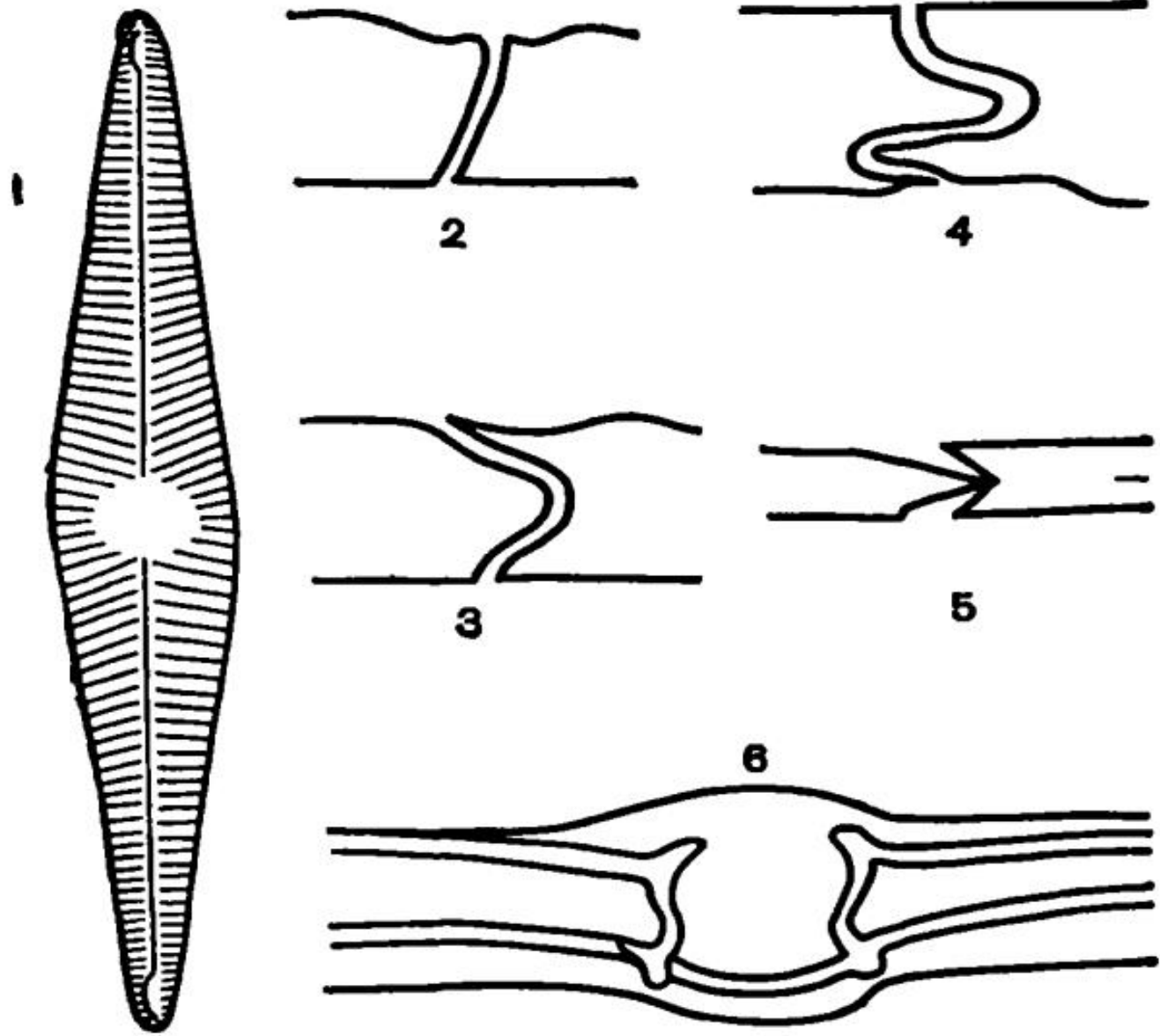
Рис. 84. Схема строения шва навiculoидного типа: 1 — створка со щелевидным швом, 2—5 — поперечный разрез щели шва, 6 — продольный разрез центрального узелка.
