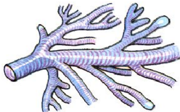
ТРАХЕИ
