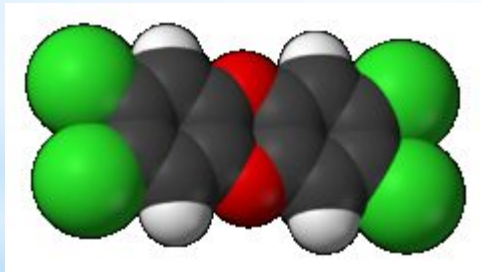
Объемная модель диоксина
