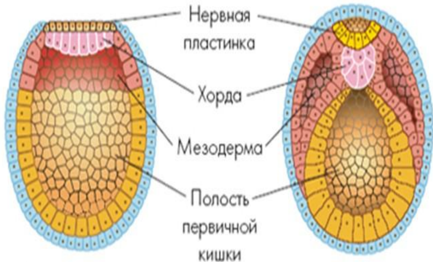
Ранняя нейрула
