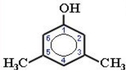
3,5-диметилфенол
