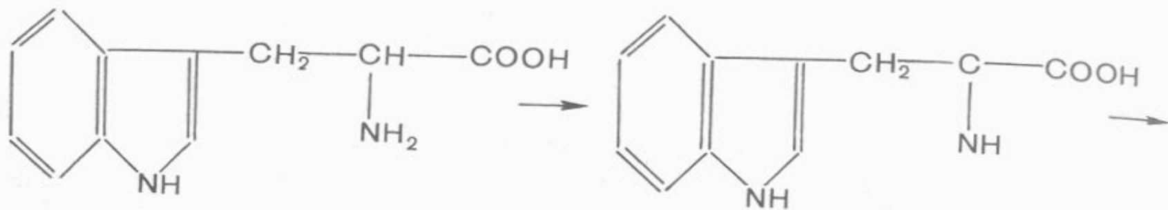
Триптофан
