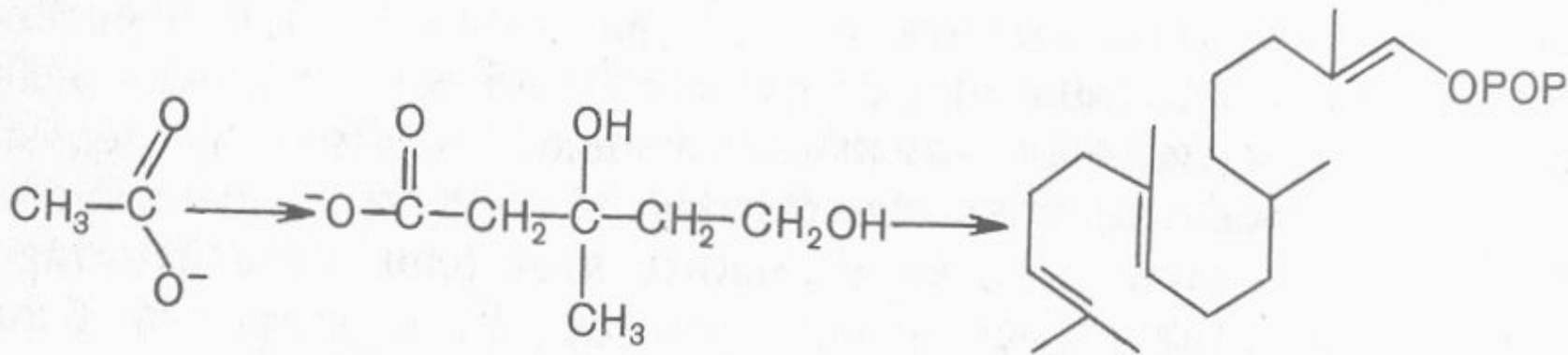
Геранил-гераниол-пирофосфат
