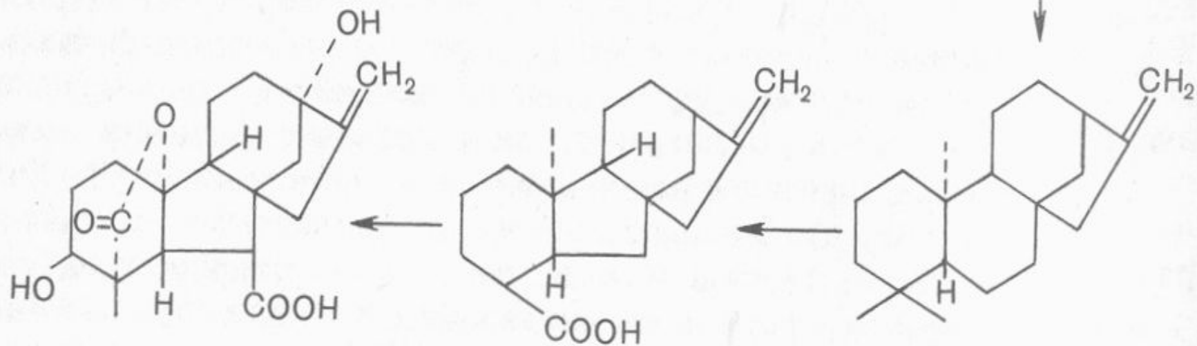
\text{C}_{10} -гиббереллины ( \text{A}_3 )
