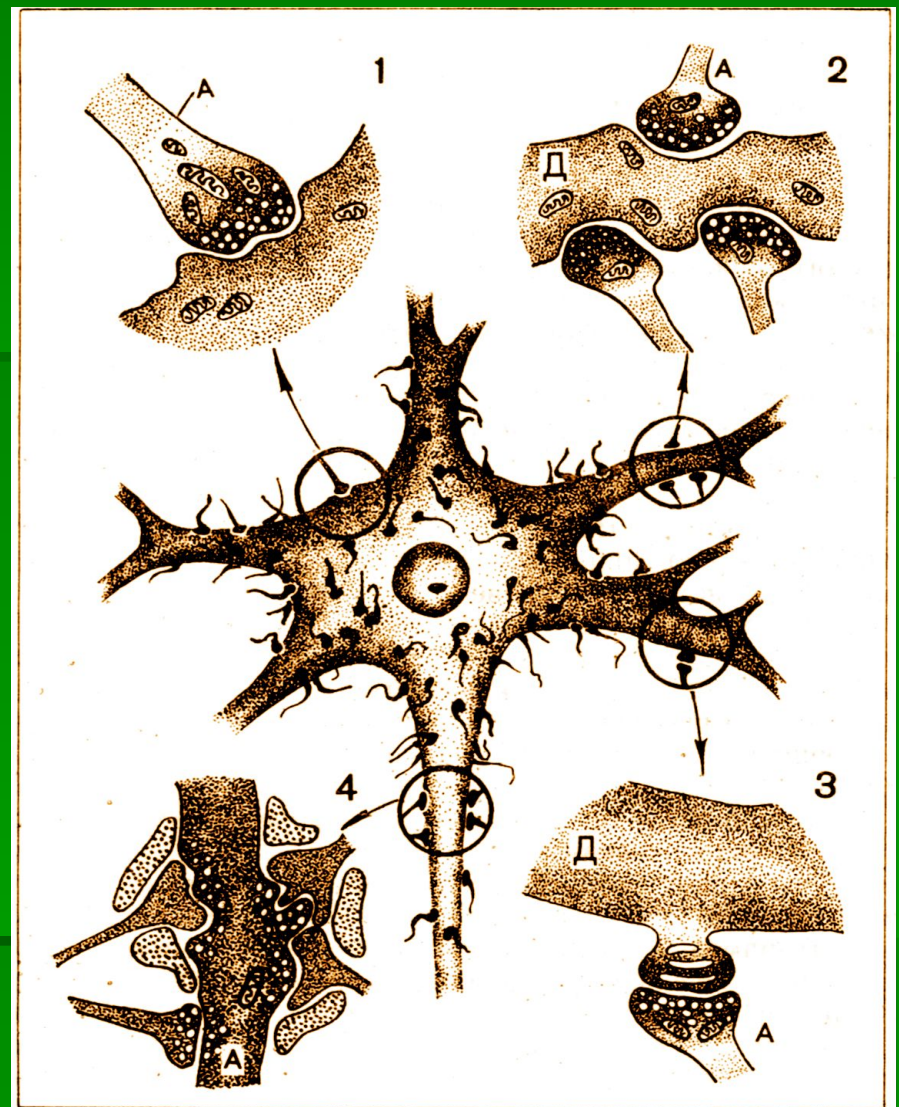
Рис. 4. Межнейронные синапсы
