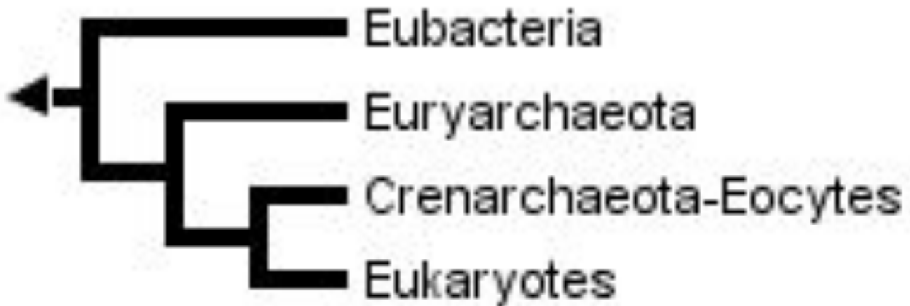
Еоцитне древо життя
