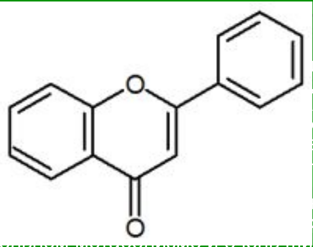
Структура флавонов
