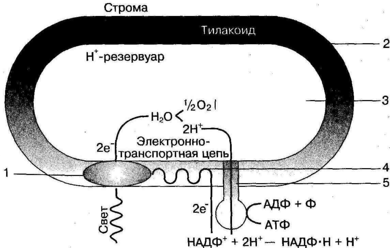
Рис. 11. Общая схема процессов световой фазы фотосинтеза, протекающих в тилакоиде: 1 — хлорофилл; 2 — мембрана тилакоида; 3 — внутренняя часть тилакоида; 4 — цепь электропереноса ферментов; 5 — канал с ферментом АТФ-синтетазой
