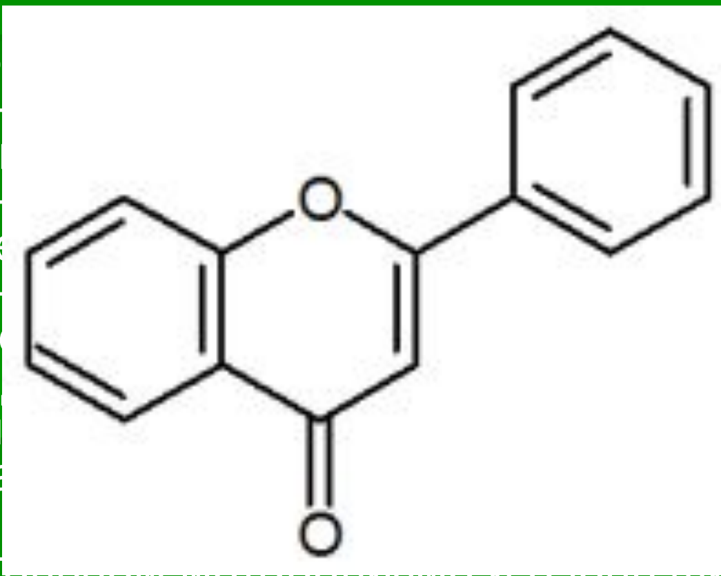
Структура флавононов
