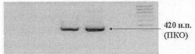
Образец гель-электрофореза
