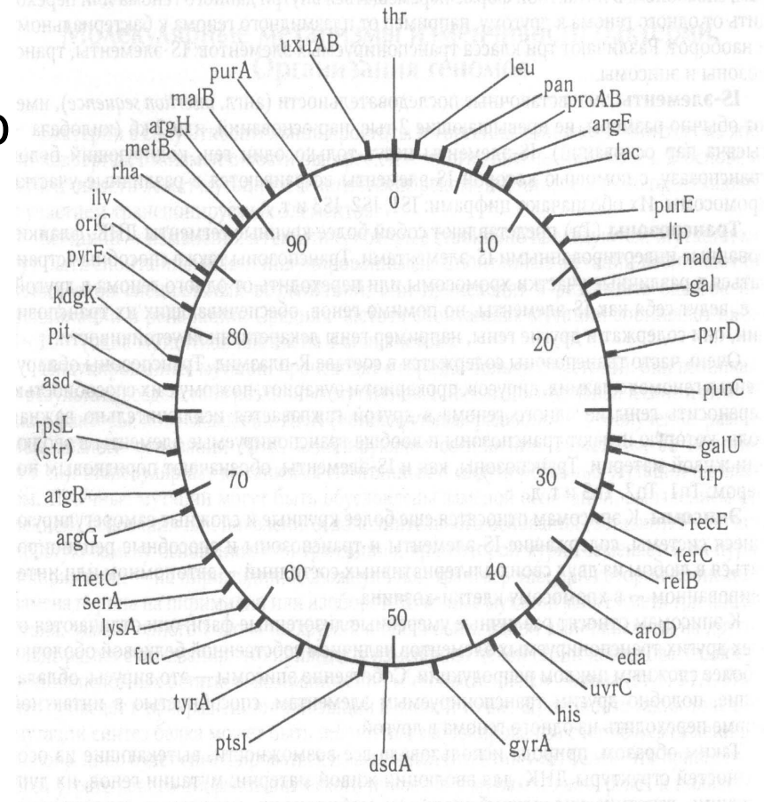
Сокращенная хромосомная карта E.coli
