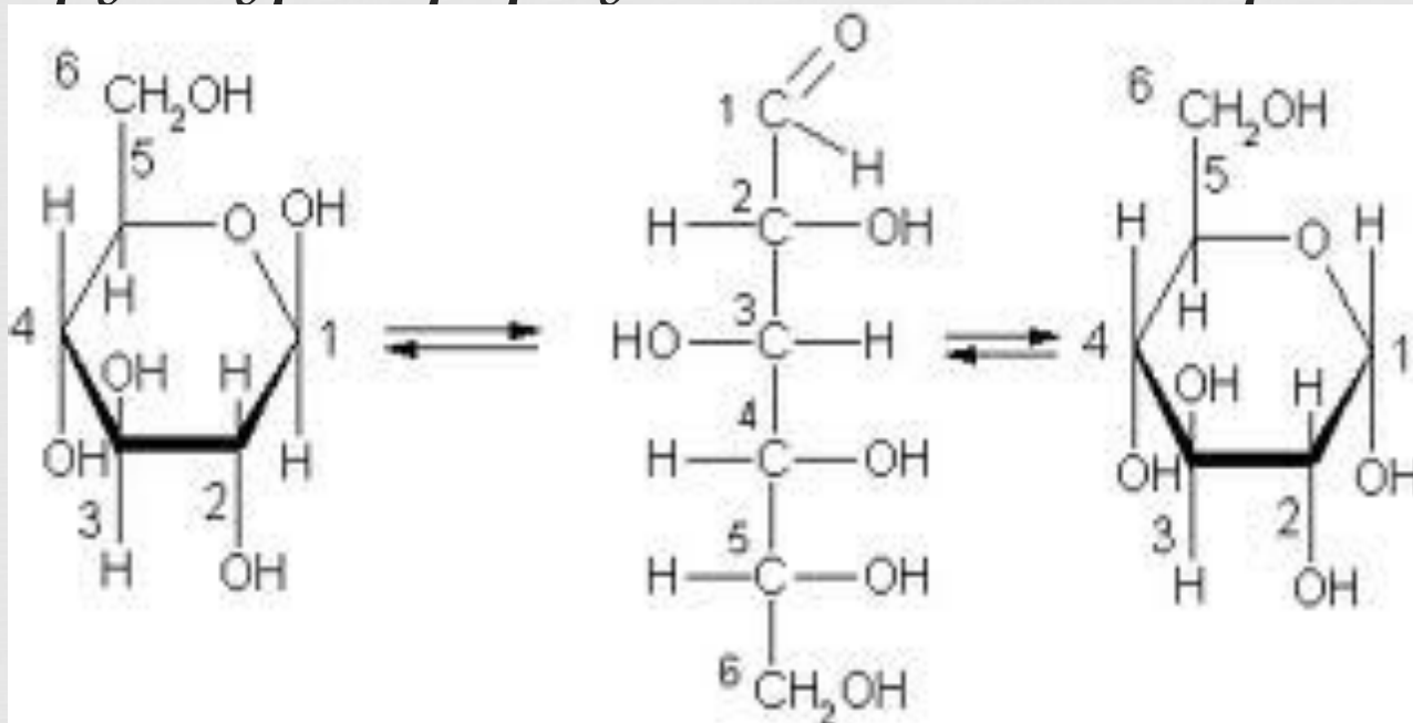
\beta -циклоглюкоза
