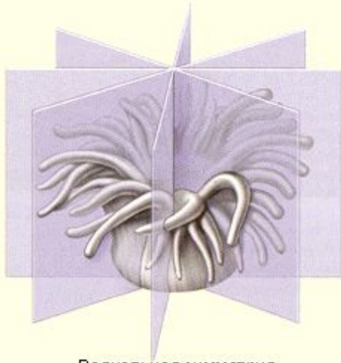
Радиальная симметрия
