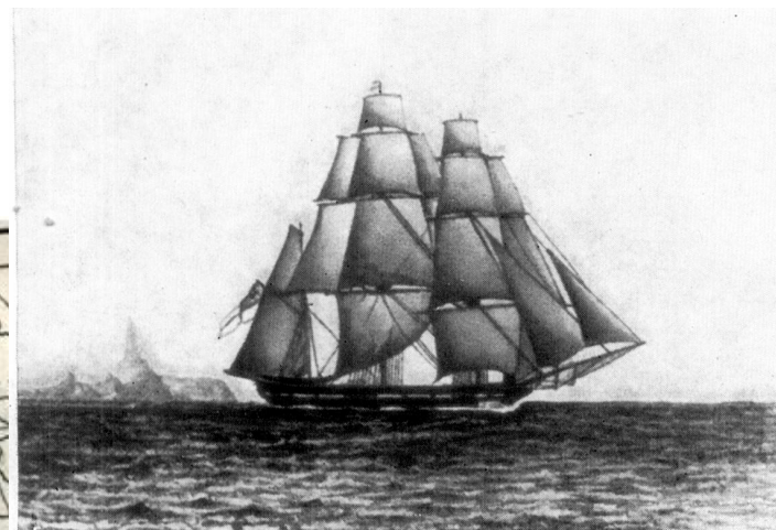
Бриг «Бигль».
