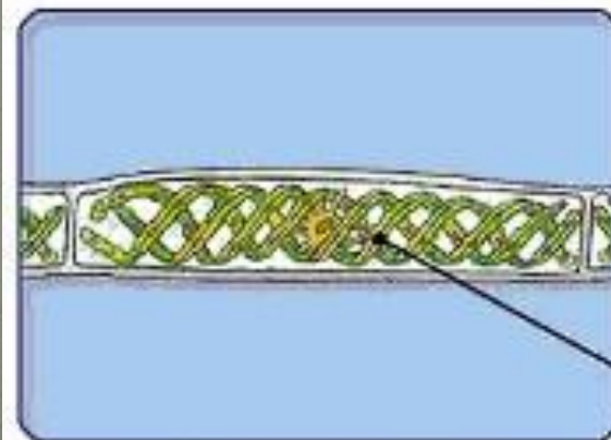
Клетка спирогиры
