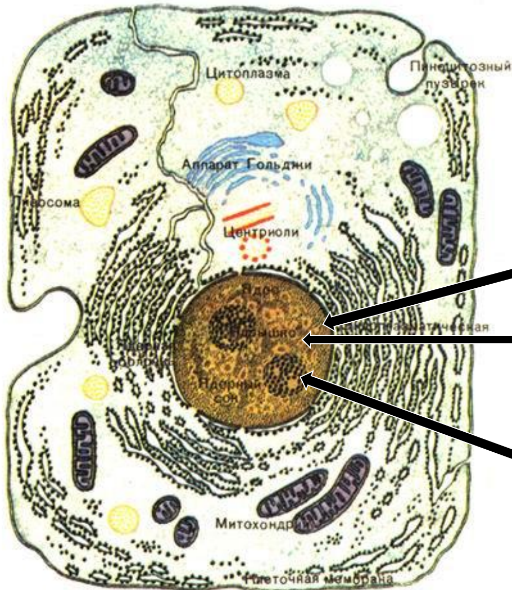
Схема строения клетки по данным электронного микроскопа.
