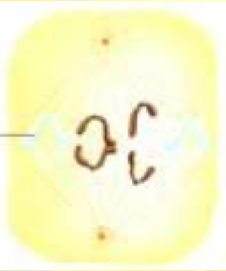
Начало анафазы
