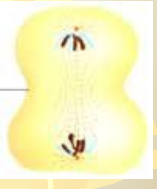
Конец анафазы
