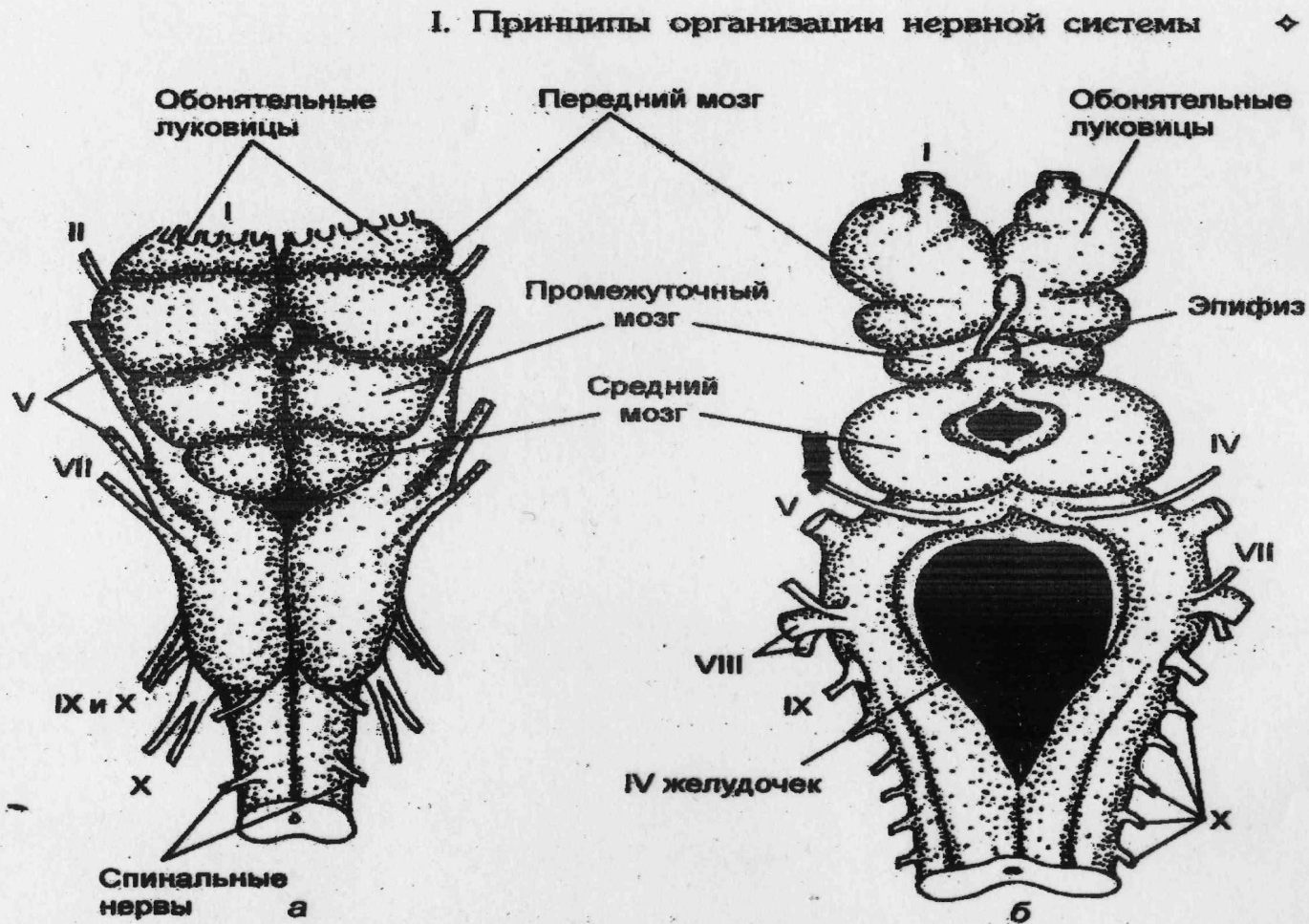
Рис. 21. Строение головного мозга миксины (а, Murchie glutinosa ) и миноги (б, Lampetra fluviatilis ). Вид с дорсальной поверхности.
