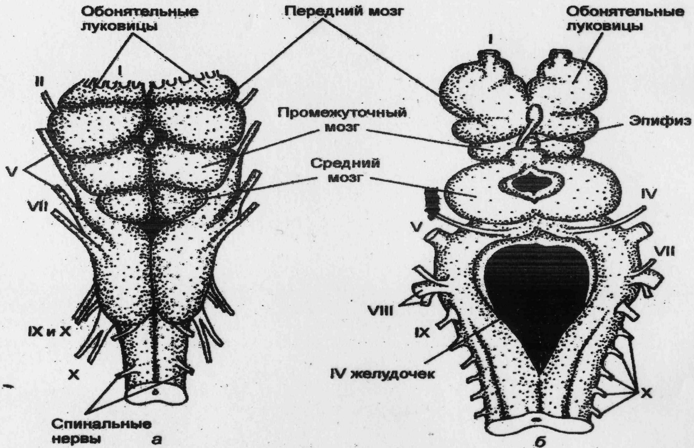
Рис. 21. Строение головного мозга миксины (а, Murchie glutinosa ) и миноги (б, Lampetra fluviatilis ). Вид с дорсальной поверхности.
