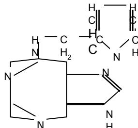
6-фурфуриламинопурин
