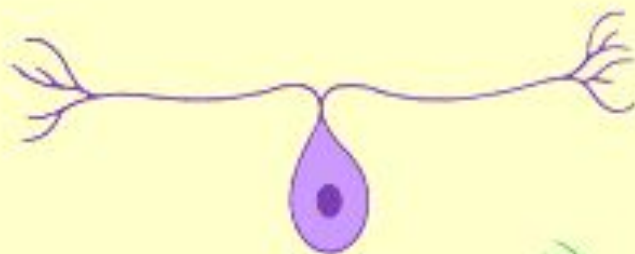
Псевдоуниполярный
