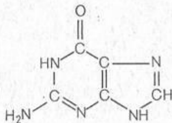
Гуанин
