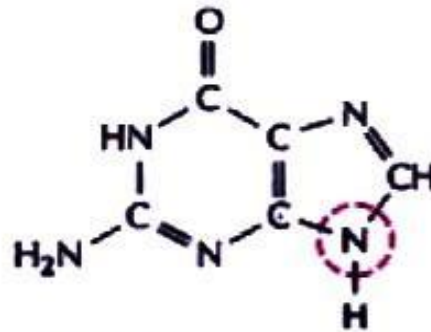
гуанин
