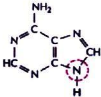
аденин
