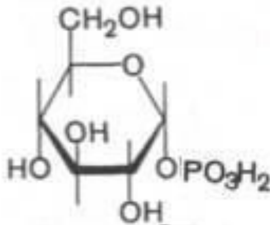
ГЛЮКОЗО-1- ФОСФАТ
