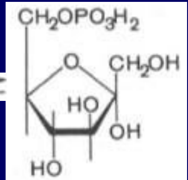
ФРУКТОЗО- 6 -ФОСФАТ
