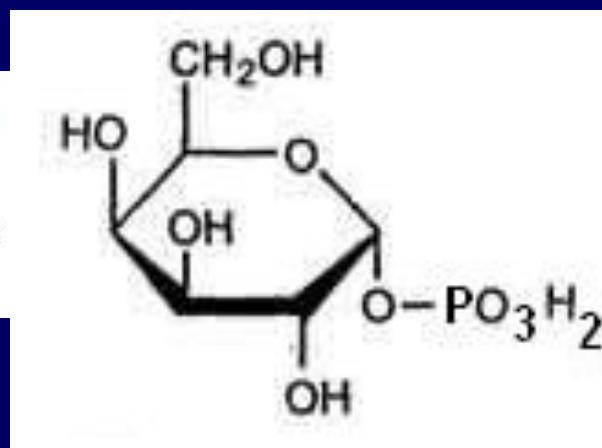
ГАЛАКТОЗО-1-ФОСФАТ
