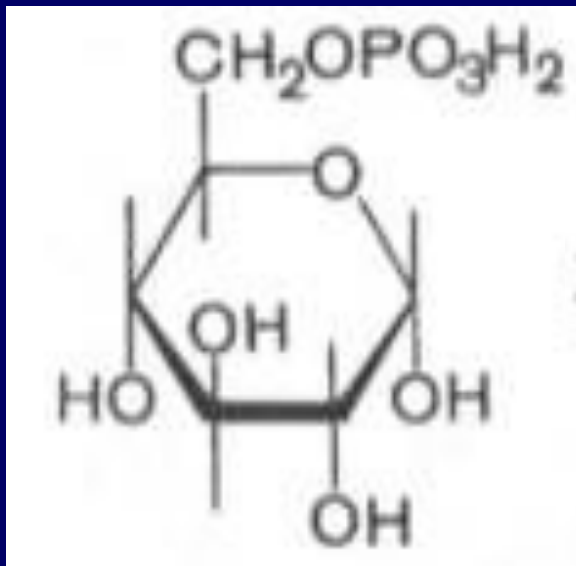
ГЛЮКОЗО- 6 -ФОСФАТ
